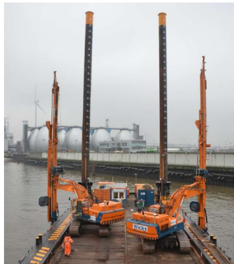
Figuur 1: voorbeeldopstelling installatie verticale drainage
